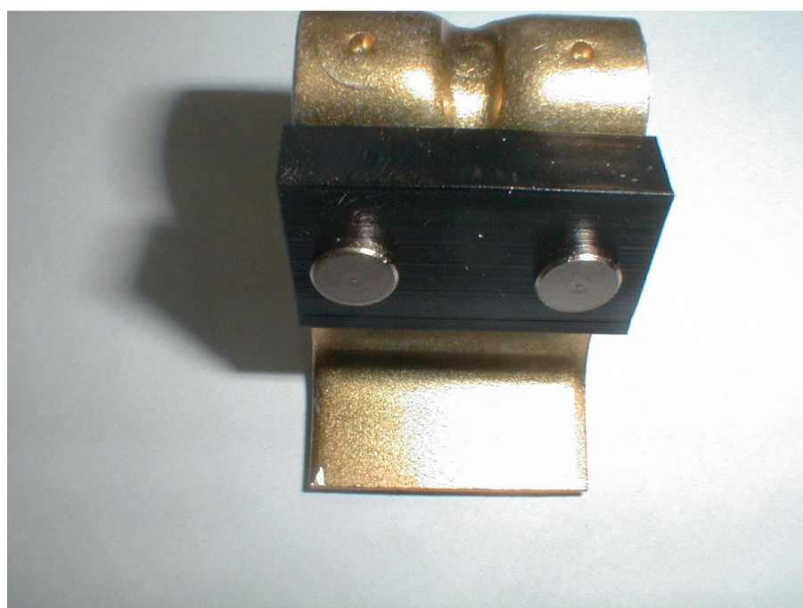
Ogranicznik ruchu styku ruchomego komory małosiejowej rozłącznika Fla 15/60 zdemontowanej po 15 latach pracy, podlega wymianie.
