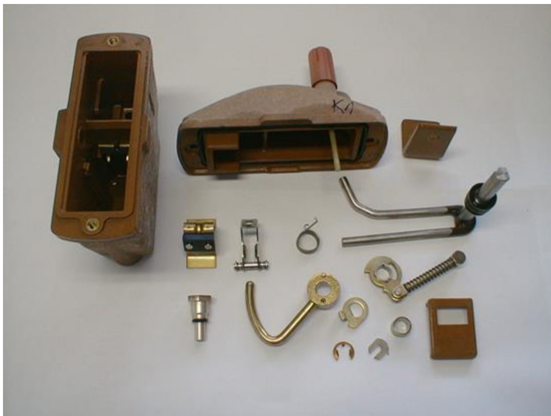
Elementy wewnętrzne komory małoolejowej rozłącznika Fla 15/60 zdemontowanej po 15 latach pracy.
