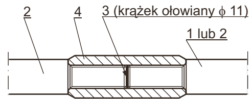
Szczegół “a”
