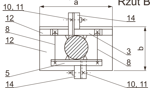
Rzut B
