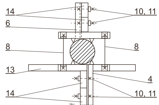
Rzut A
